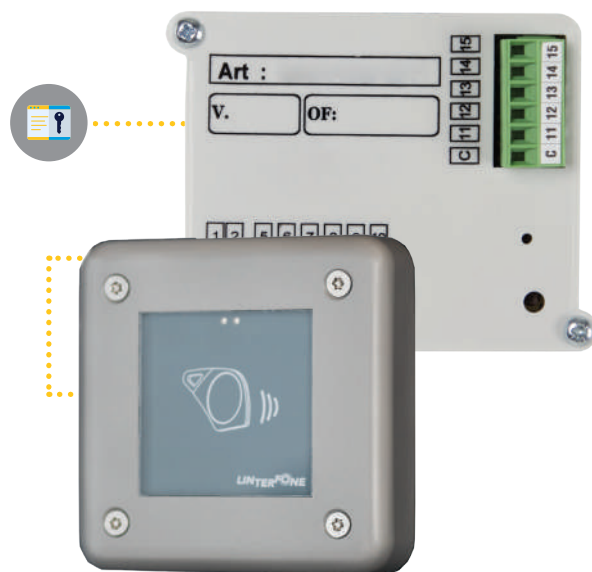
Dimensions du lecteur : 100 x 100 x 25 mm
